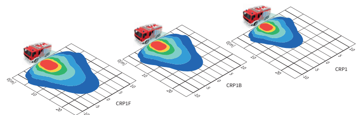
Światło o natężeniu 1 lx umożliwia czytanie tekstu w gazecie Ustawienie lampy: h=2,5m
