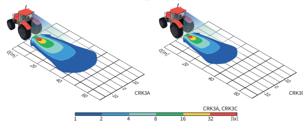
Światło o natężeniu 1 lx umożliwia czytanie tekstu w gazecie Ustawienie lampy: 8° od pionu, h=2,5m
